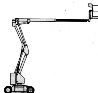
PEMP type 3B PEMP automotrice à élévation multidirectionnelle
